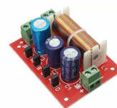
[5626]Divisor de frecuencia pasivo crossover de 2 vias 400w $15750
