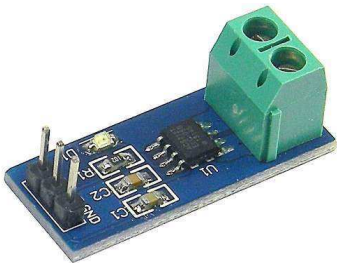
[1690]Sensor De Corriente \pm 5a Efecto Hall Acs712 Arduino Pic Avr $1799
