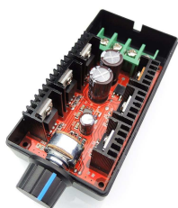
[2014]Pwm Control De Velocidad Para Motores Dc 2000w 10-50v 40a $25470
