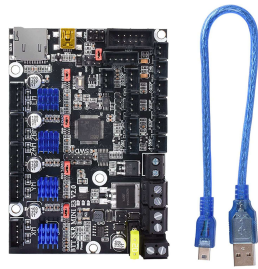
[5482]Placa Bigtree tech Skr Mini E3 V2 0 32b Tmc2209 Ender 3 Cr10 $66600
