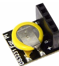
[2708] Mini Reloj Tiempo Real Rtc Ds3231 Raspberry Ard Arm Pic $5130
