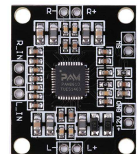
[2232]Modulo Amplificador Pam8610 2x10w 5v A 15v Arduino Clase D $2088
