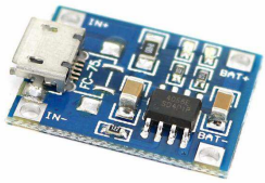
[2702]Tp4056 C/protec Cargador Bateria 18650 Micro Usb Arduino $621
