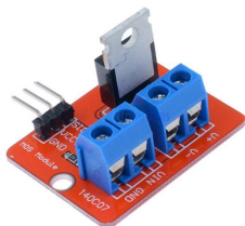
[2780]Modulo Driver Mosfet Irf520 24v 9a Controlador Arduino Pic
