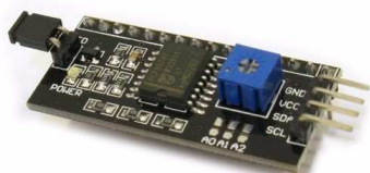
[1214]Adaptador Paralelo-serie I2c Mps Entradas En Tu Arduino Lcd
