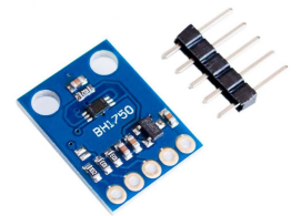
[4175]Modulo Sensor Digital Luz Ambiente Lux Bh1750 Arduino $3780
