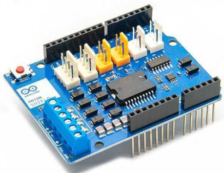
[2648] Shield ARDUINO control de motores L298p 2.0 2 motores CC
