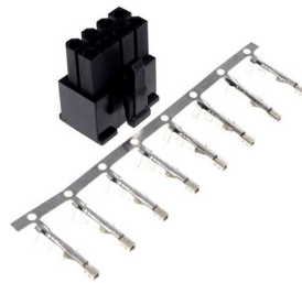
[5060]Ficha Conector Macho de 4,2mm GPU PCI-E con 8 pines
