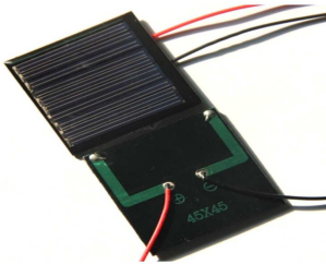
[5984]Panel Solar Celda Solar Con Cable 0.25w 5v 45x45mm Arduino
