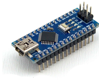
[2593]Arduino Nano V3.0 Atmega328p Ch340g 16m 5v Con pines soldados
