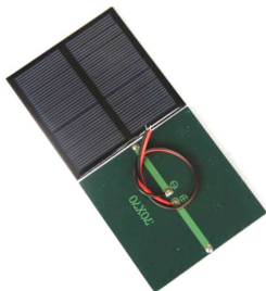
[5992]Panel Solar Celda Solar Con Cable 0.7w 1.5v 70x70mm Arduino
