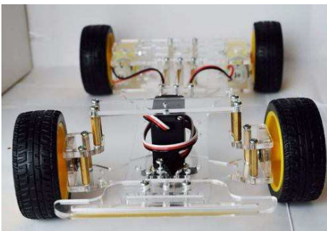
[1758]Chasis Para Armar Auto Inteligente 4w Arduino + Servo S3003
