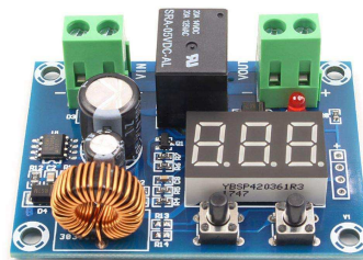
[2962]Modulo de protección de voltaje XH-M609 24V DC 12V
