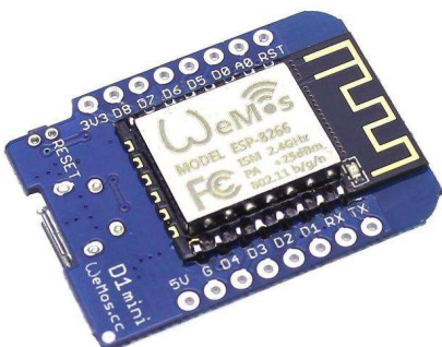
[2446]Modulo Nodemcu Wemos D1 Mini Wifi Esp8266 Esp12f 4mb Arduino
