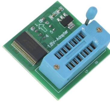
[5345]Adaptador 1.8 V Spi Flash W25 Mx25 Ch341a Ezp2013 iPhone
