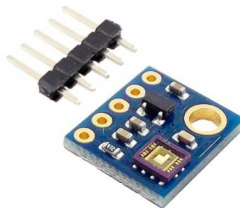
[5478]Modulo Sensor Latidos Arduino Cardio Finger Heartbeat Ultravioleta Uv MI8511 Arduino
