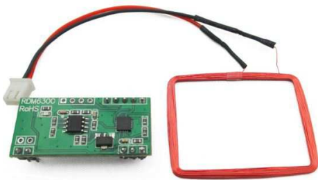
[1799]Rfid Rdm6300 Lector De Tarjetas Tags Tokens 125khz Uart
