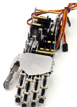
[4571]Kit Para Armar Robot Mano Robotica Derecha Con 5 Dedos Servo
