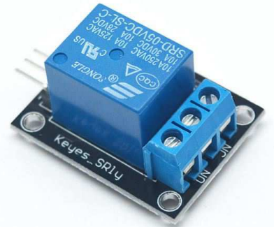
[1204]Modulo Rele 5v Simple Inversor Contactos De 10a 220v Arduino
