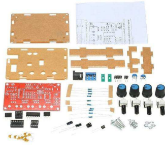
[4600]Generador De Señales De Función Icl8038 Diy 5hz-400khz
