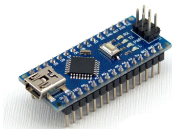
[2593]Arduino Nano V3.0 Atmega328p Ch340g 16m 5v Con pines soldados
