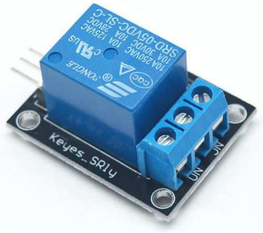
[1204]Modulo Rele 5v Simple Inversor Contactos De 10a 220v Arduino
