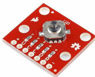
[1533]Modulo Adaptador Interruptor Tactil De 5 Vias Arduino
