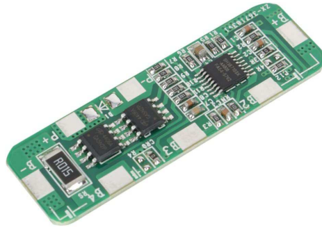
[1937]Modulo Placa Protección cargador 3 baterias 18650 12.6V 10a
