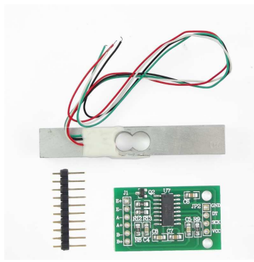
[2783]Celda 10KG De Carga Con Amplificador Hx711 Arduino
