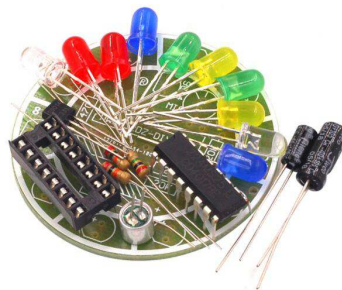
[4731]Kit Para Armar Juego Luces Led Giratoria Activados Por Voz
