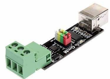
[1373]Modulo Adaptador Usb A Rs485 / Rs422 Con Ft232r1 Y Max485
