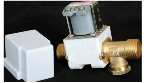
[2471]Valvula Electrica Para Liquidos 12v De 1/2 Arduino, Pic
