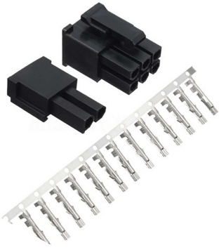
[4809] Conector Pci Express De Alimentación 8pin Hembra Atx Eps 6+2
