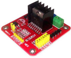
[1811]Doble Puente H Driver L298n Motor Dc Arduino Arm Avr L298
