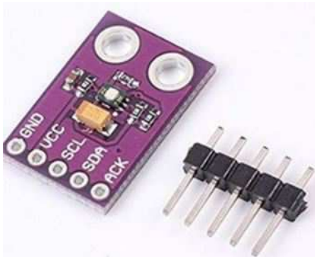
[1946]Modulo Sensor Detector Ultravioleta Veml6070 Arduino
