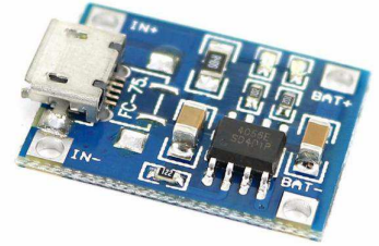
[2702]Tp4056 C/protec Cargador Bateria 18650 Micro Usb Arduino
