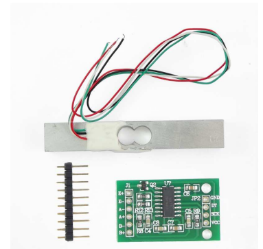
[2783] Celda 10KG De Carga Con Amplificador Hx711 Arduino
