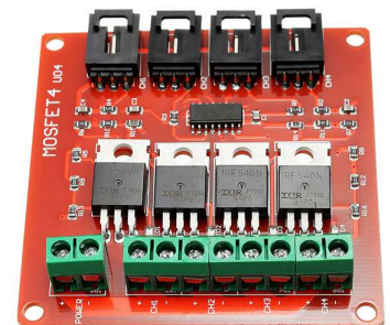
[2694]Módulo De Interruptor De 4 Canales Mosfet 4 Route Button
