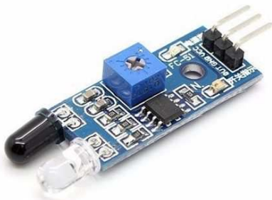
[1581]Modulo Detector Sensor De Obstaculos Infrarrojo Arduino Pic
