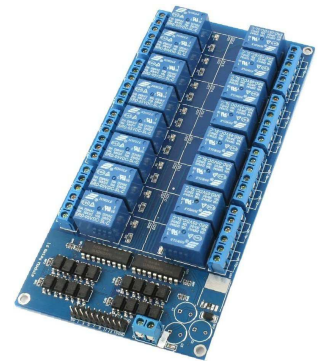
[1207]Modulo De Relee Relay Opto 16 Canales 5V Arduino Dsp Avr
