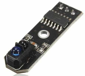
[1767]Sensor Infrarrojo Seguidor De Linea Tracker Ir Tcrt5000
