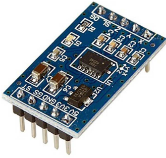
[1367]Acelerometro Mma7361 3 Ejes Sensor Inclinacion Xyz Arduino
