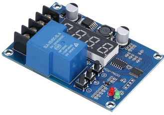
[5457]Modulo Control Carga Baterias Lito 6-60v 12-24v 30a Xh-m600
