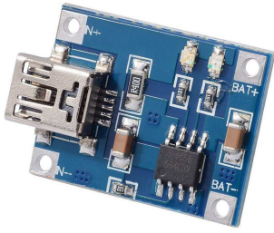
[2278]Modulo De Carga Micro Usb 5v 1a 18650 Tp4056 Bateria Litio
