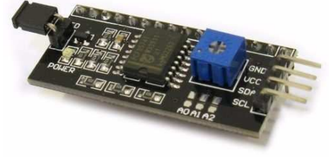
[1214]Adaptador Paralelo-serie I2c M 2 s Entradas En Tu Arduino Lcd
