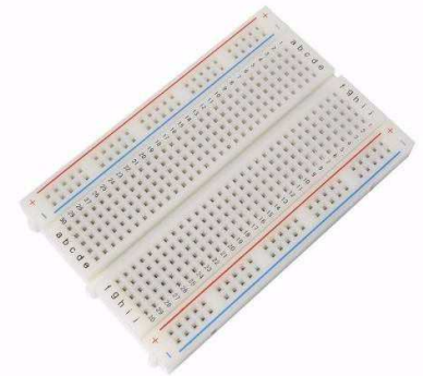
[1343]Protoboard De 400 Puntos Experimentador Arduino Breadboard
