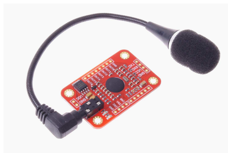
[2001]Modulo de Reconocimiento De Voz + Microfono Arduino Voice
