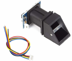
[2277]Modulo De Identifiacion De Huella Dactilar Uart Arduino
