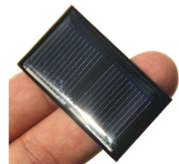
[5950]Modulo Mini Panel Solar Policristalino 1v 125ma 45x25mm
