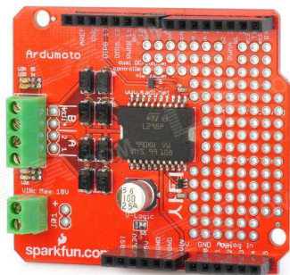
[2579]Ardumoto Motor Driver Shield L298p 2a Dual Dc Arduino X Aa con Plug conexion Arduino
