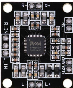
[2232]Modulo Amplificador Pam8610 2x10w 5v A 15v Arduino Clase D
