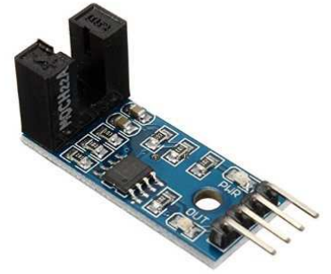
[2303]Sensor Optico Horquilla Velocidad Tacometro Lm393 Arduino
