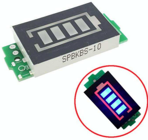
[2985]Modulo Indicador Carga De Bateria De Litio 3s 11.1v - 12.6v
