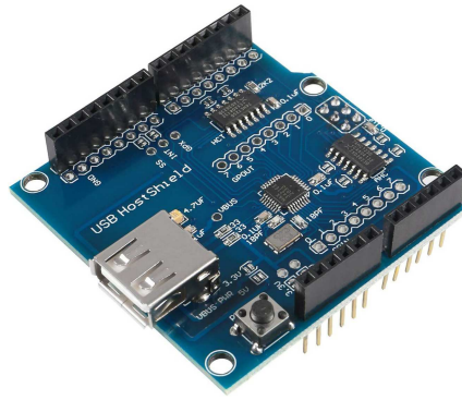
[2364]Host Usb Adk Shield Arduino Uno Mega Leonardo Usa Android
