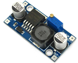
[1965]Lm2596 Fuente Step Down Dc-dc Ajustable 1.25v 35v 3a Arduino
