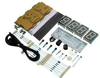
[2906]Kit Para Armar Reloj Digital 4 Digitos Inteligente Led Color
