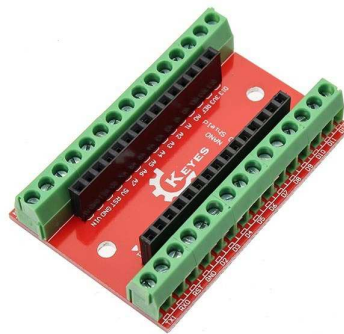
[2806]Arduino Nano Shield V3 Con Borneras Screw Placa De Expansion
