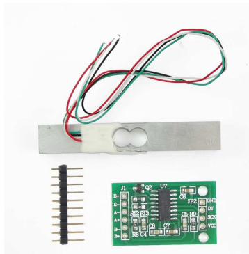
[2781]Celda De Carga 1kg Con Amplificador Hx711 Arduino
